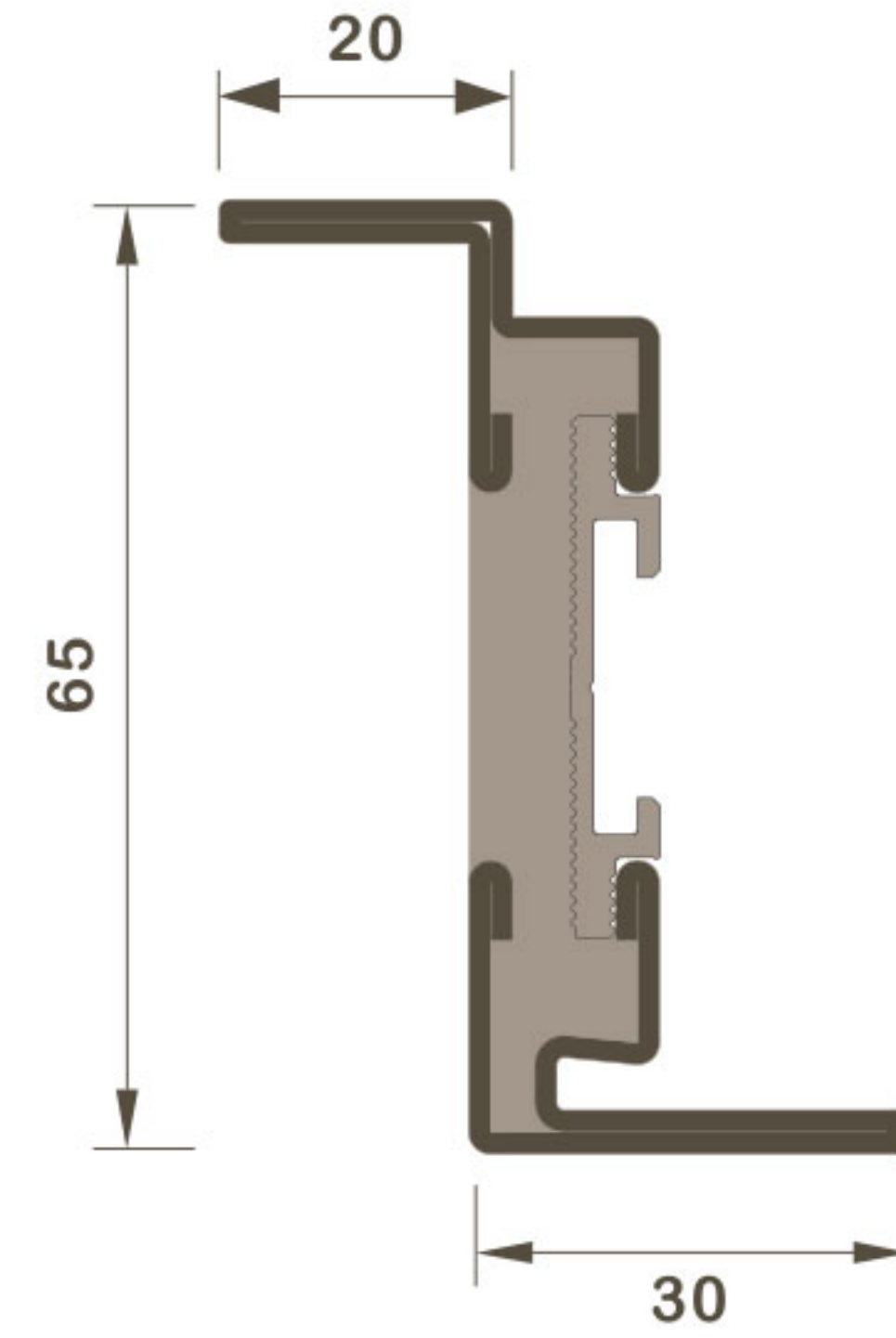
S-X02 Gfe : 2.91kg/m O : 0.18m 2 /m
