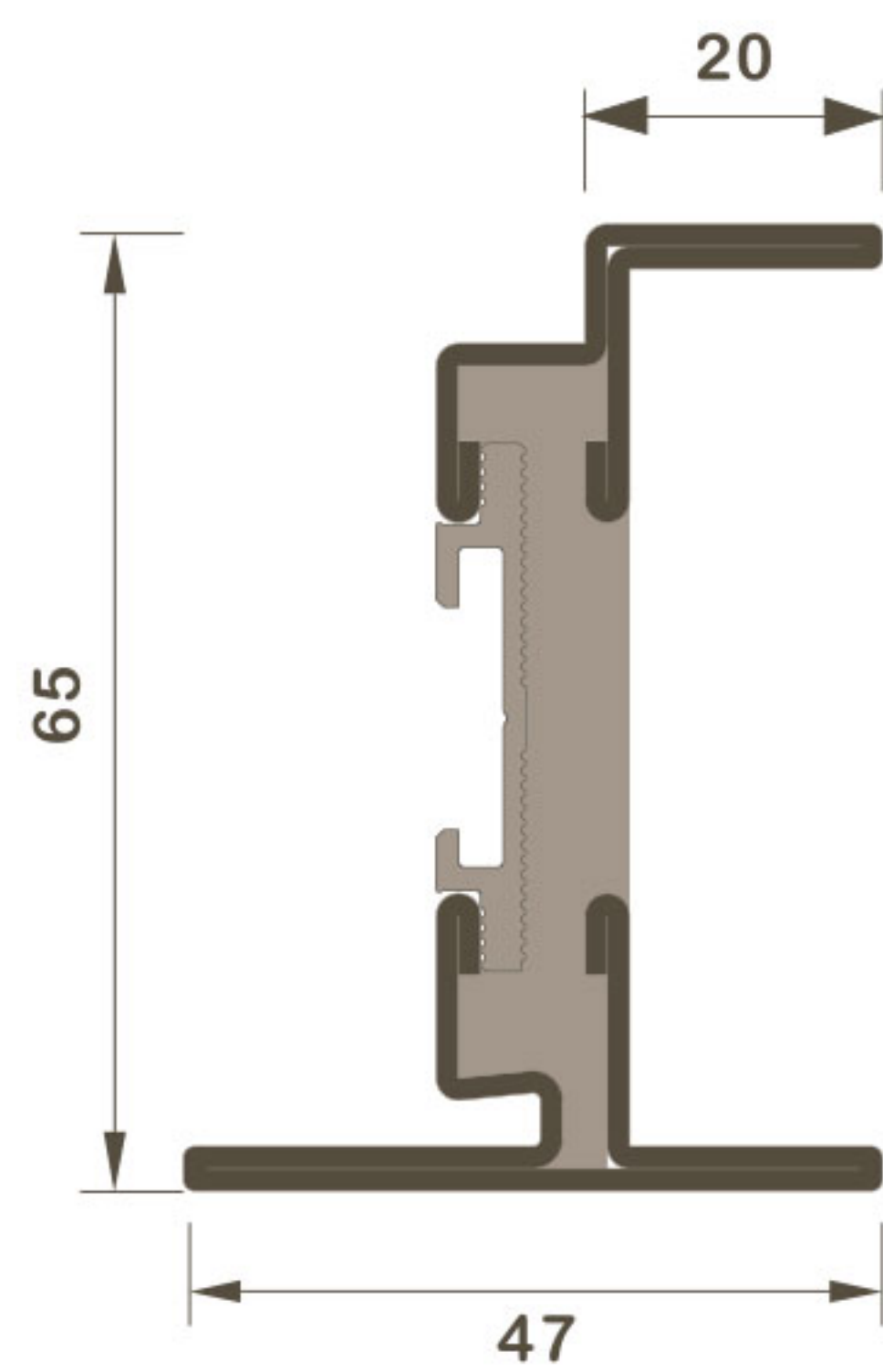
S-X09 Gfe : 3.3kg/m O : 0.21m 2 /m
