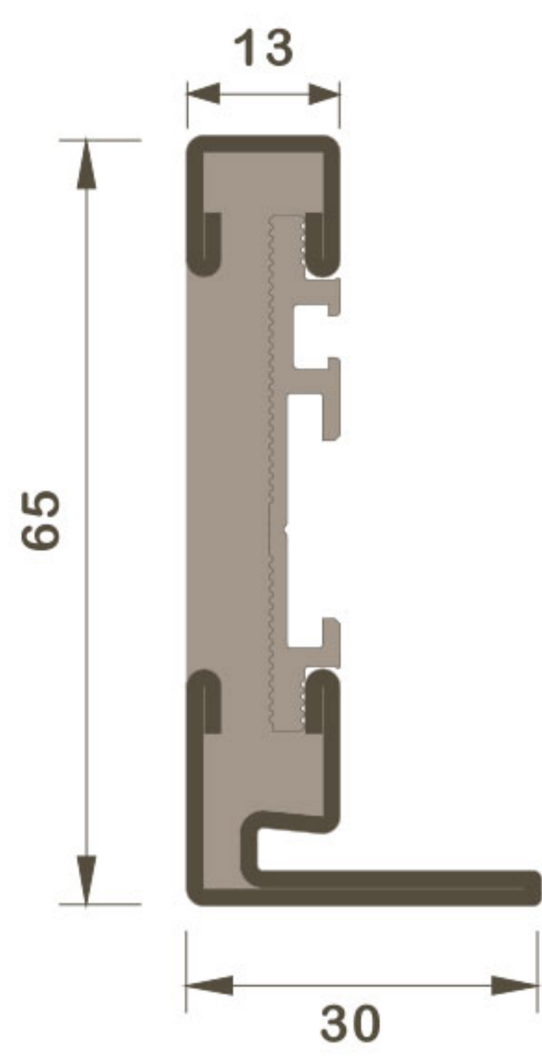
S-X08 Gfe : 2.31kg/m O : 0.14m 2 /m
