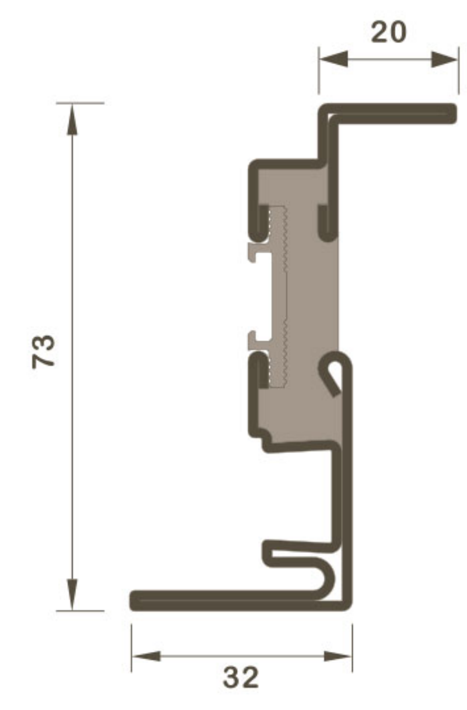
S-X013 Gfe : 3.67kg/m O : 0.2m 2 /m
