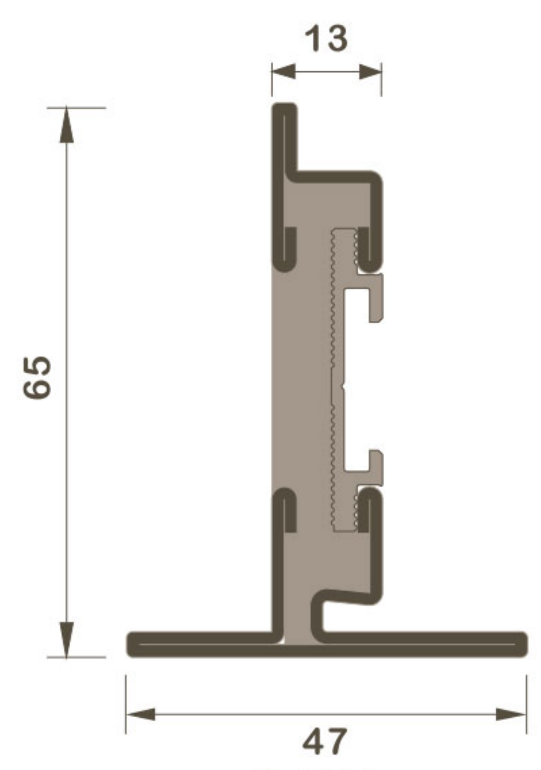
S-X03 Gfe : 2.86kg/m O : 0.17m 2 /m
