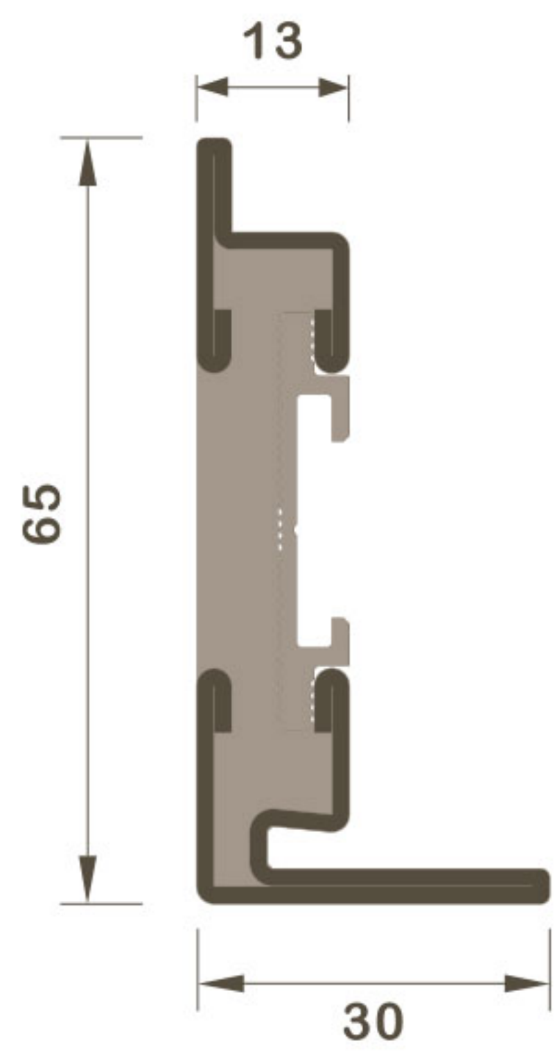
S-X01 Gfe : 2.47kg/m O : 0.14m 2 /m
