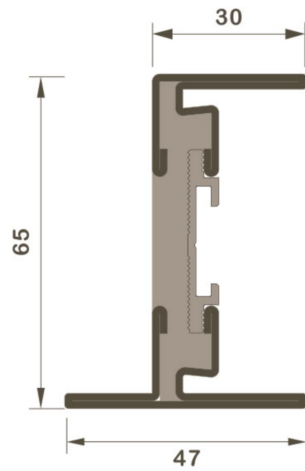
S-X04 Gfe : 3.42kg/m O : 0.21m 2 /m
