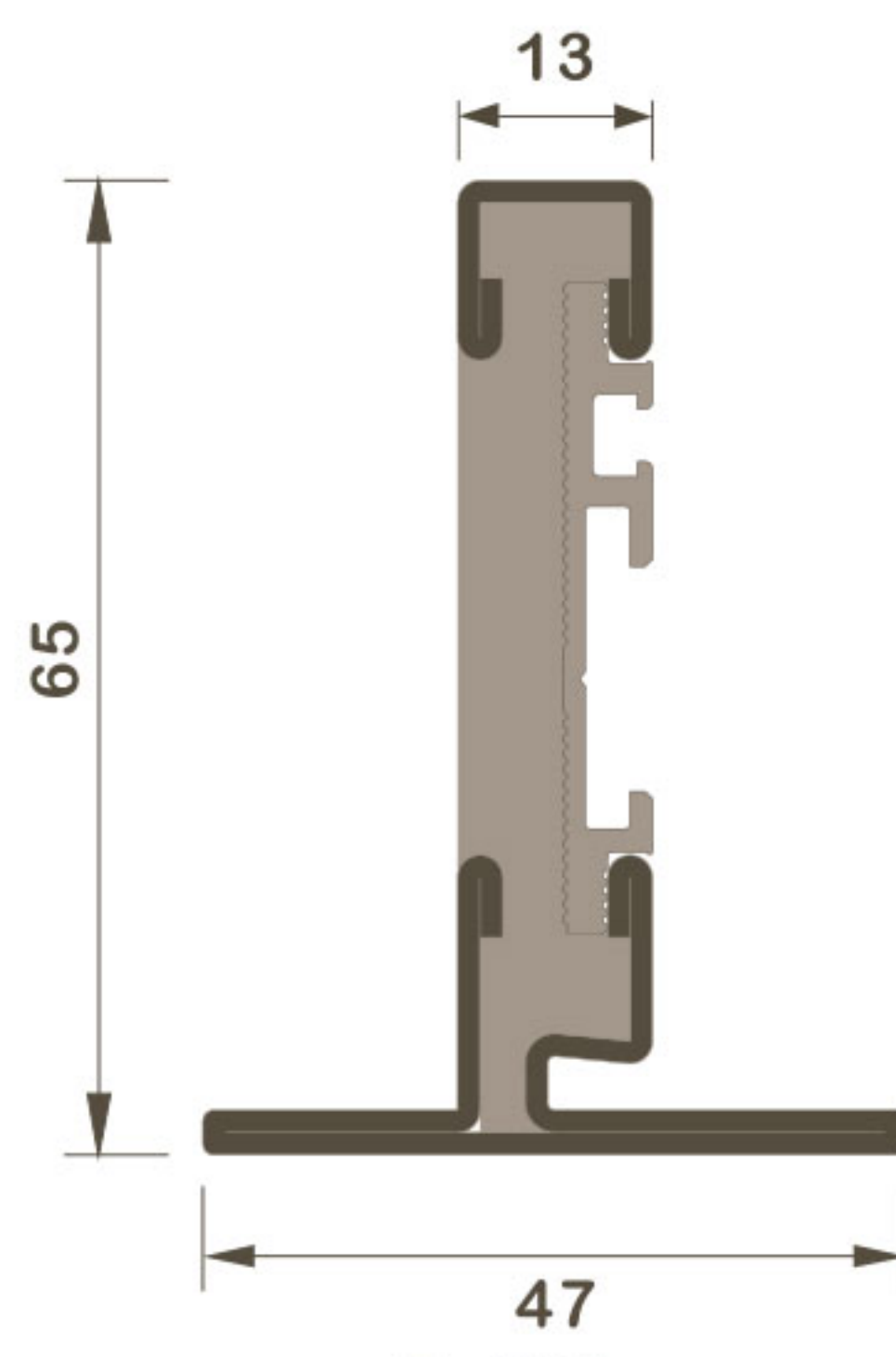
S-X05 Gfe : 2.7kg/m O : 0.17m 2 /m
